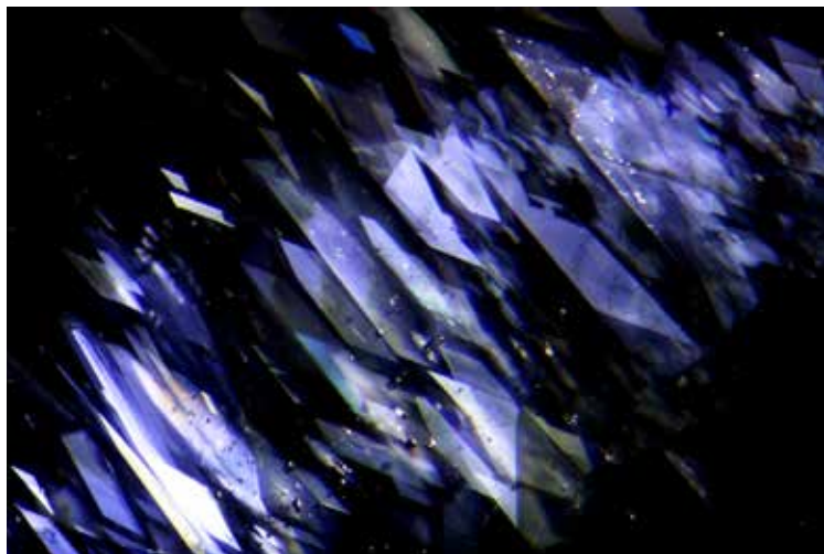
Höbomit-Lamellen in Kobaltspinell aus Tasnsania
